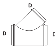
TES SIMPLES 45°
